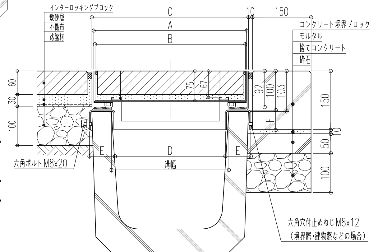
施工参考図
